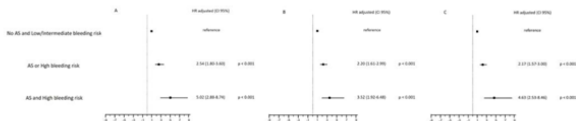
Figura 2. Hazard ratio ajustados para la asociación entre el score combinado y el sangrado mayor a 18 meses de seguimiento. El score combinado incluye la función valvular aórtica y las categorías de riesgo hemorrágico. A) HAS-BLED, B) ATRIA y C) ORBIT.
