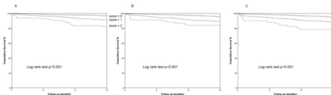
Figura 1. Curvas de supervivencia Kaplan-Meier para sangrado mayor en función del score
